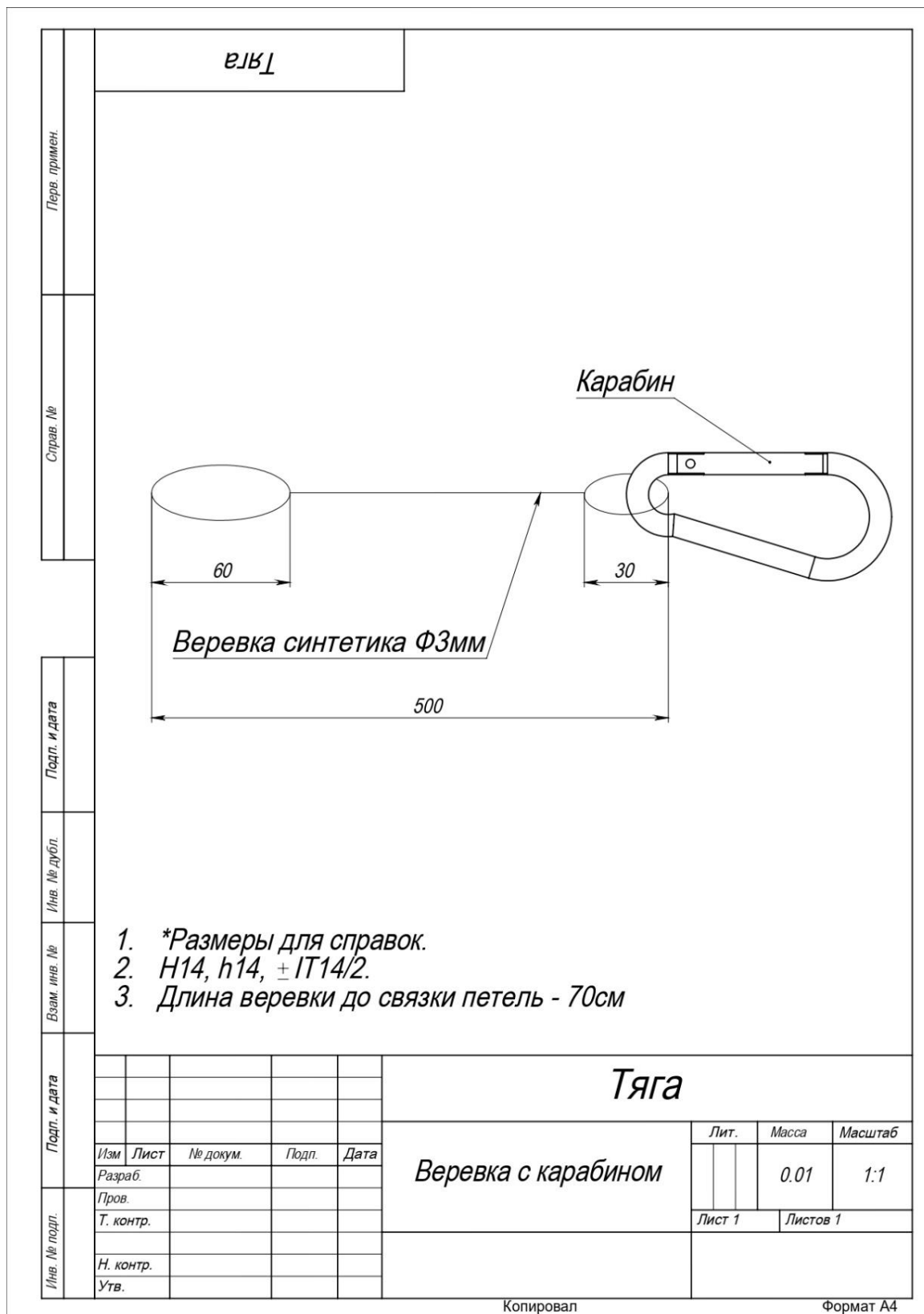
Рисунок 7. Тяга
