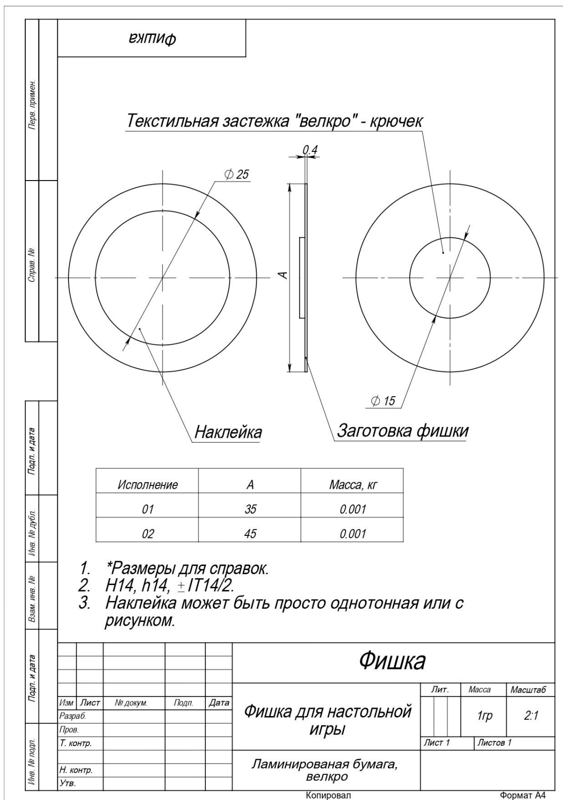
Рисунок 9. Фишка
