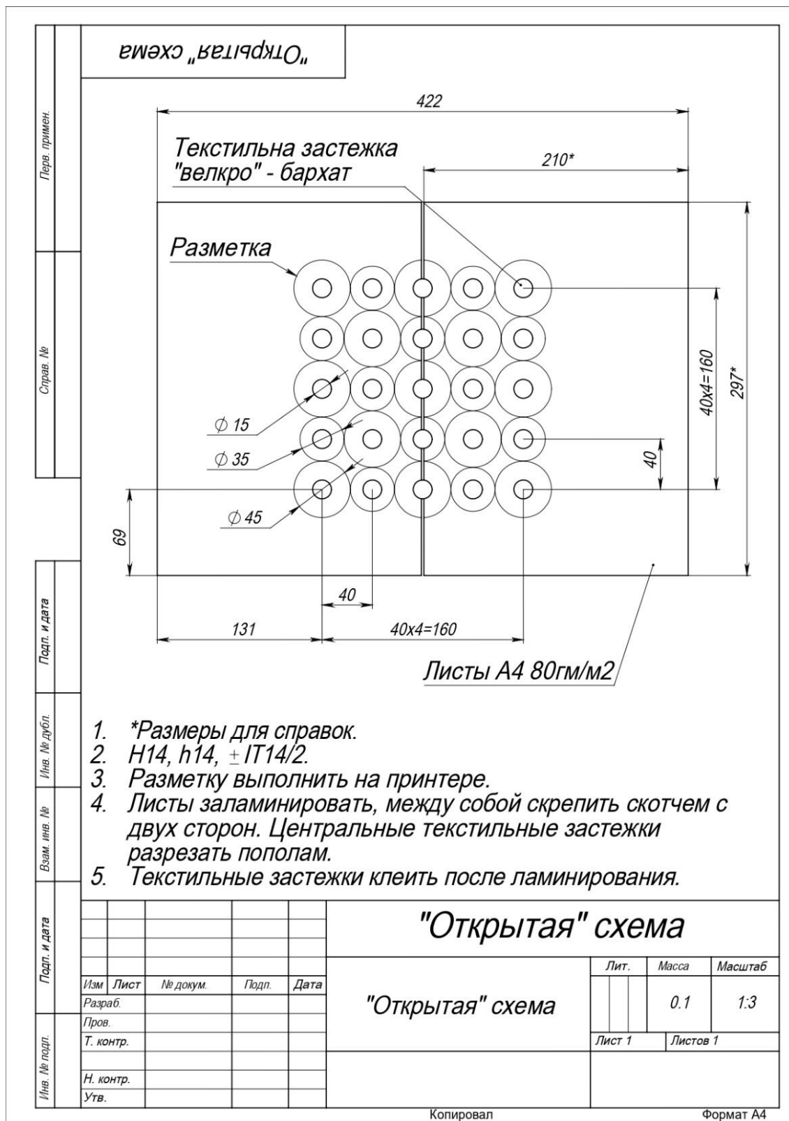
Рисунок 8. «Открытая» схема
